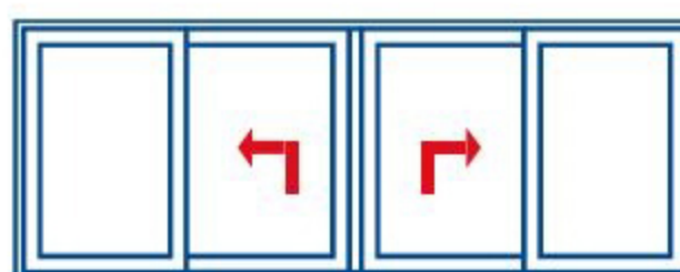
Porta 4 ante con 2 ante alzante-scorrevoli e 2 ante fisse
